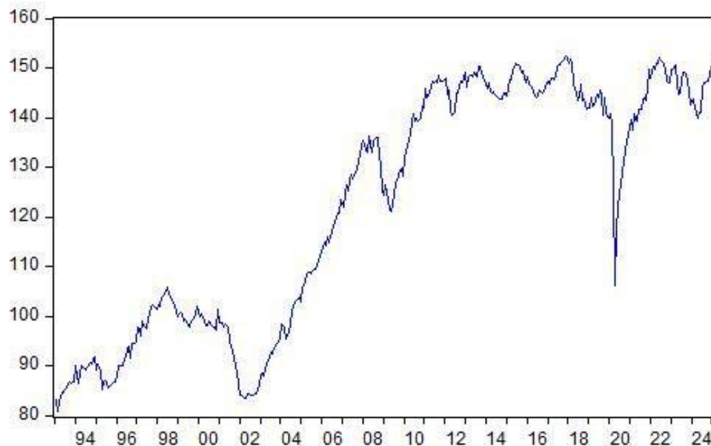
EMAE
